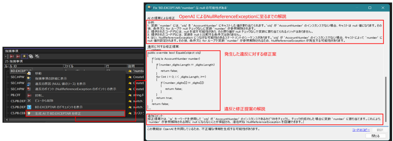
図 1：OpenAI 機能を活用した違反修正のイメージ
