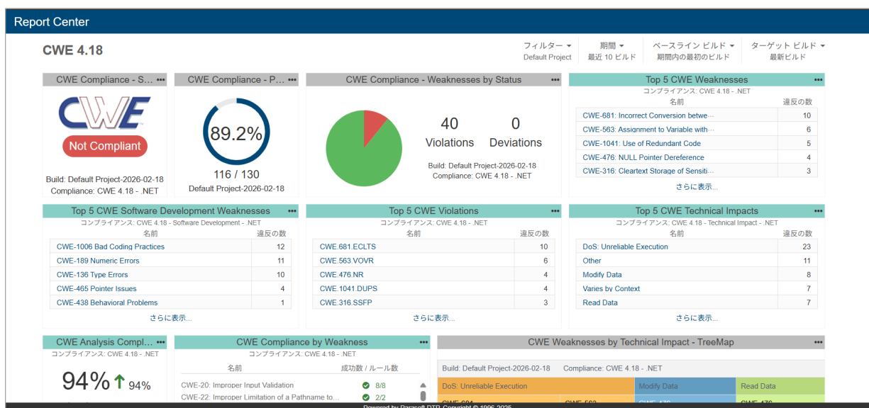
図5：CWE4.18用ダッシュボードイメージ
