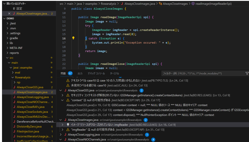
図 2: Visual Studio Code の静的解析結果の確認イメージ
