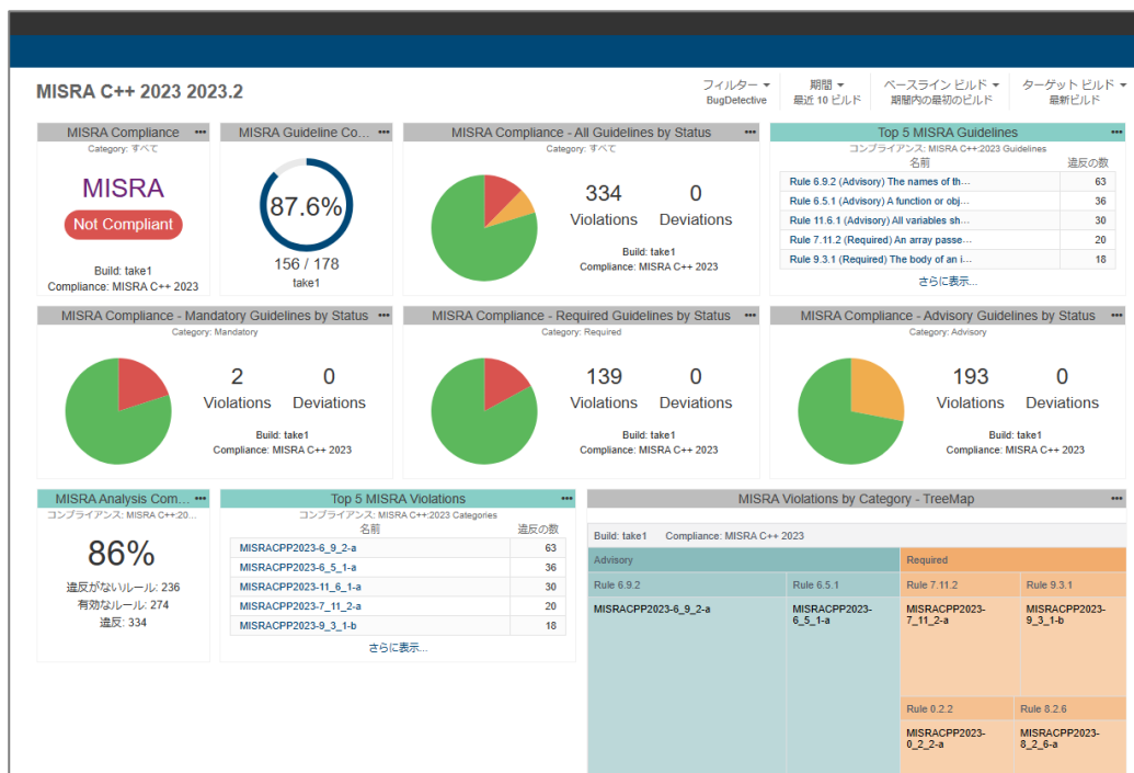
図 1. Parasoft DTP における MISRA C++:2023 ダッシュボード
