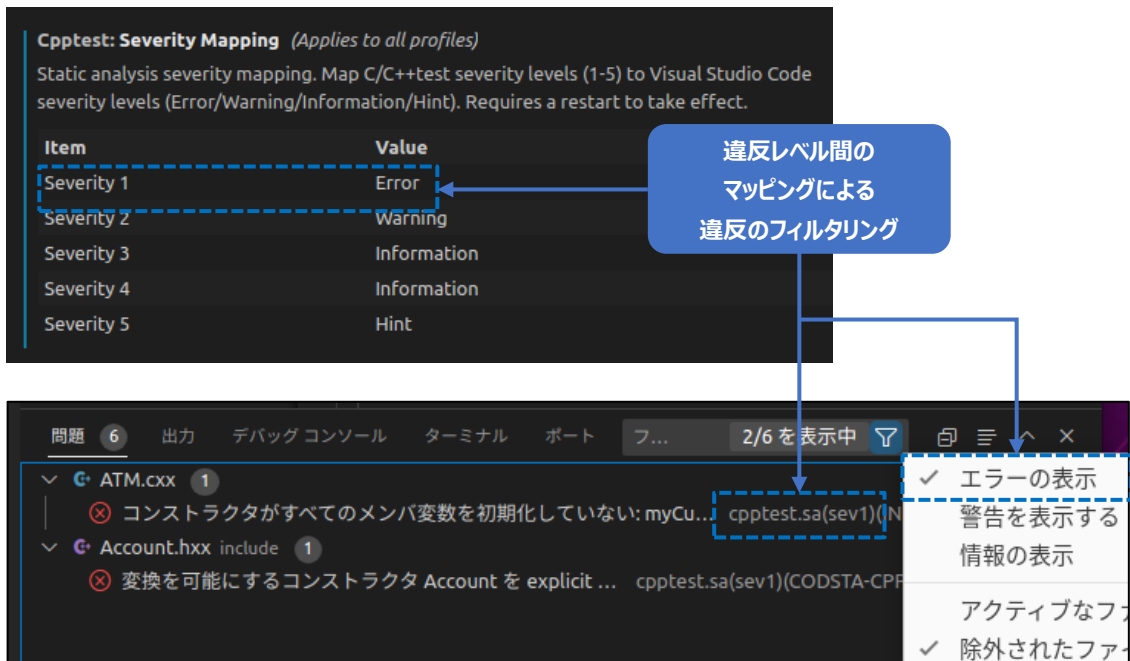
図 3. VS Code のコード診断機能との連携
